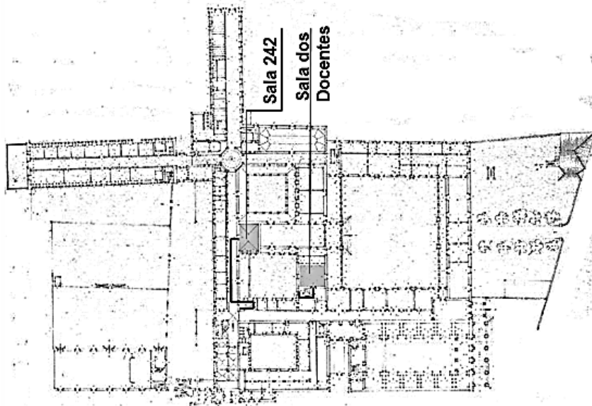
COLÉGIO DO ESPÍRITO SANTO PLANTA BAIXA - PISO 2
